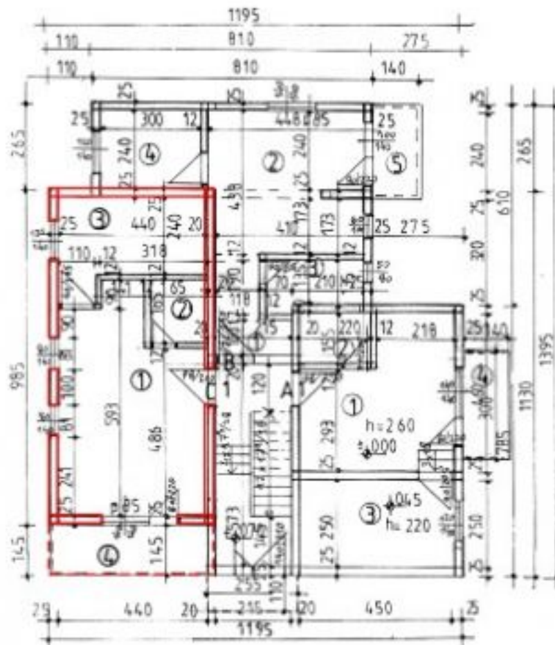
OSNOVA R 1:100
